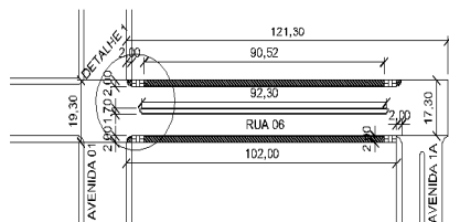
LAYOUT ÁREA A SER PAVIMENTADA Unidade: m Escala 1/1.000
